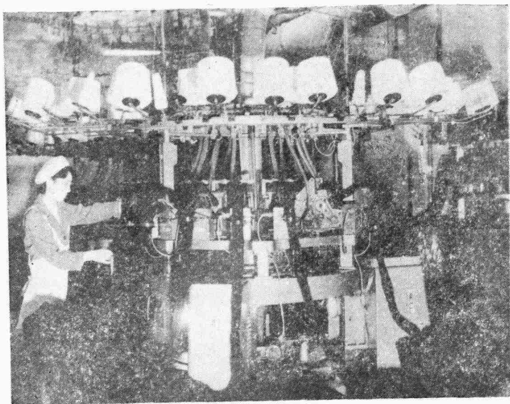
无锡市人造毛皮厂1985年引进的电子提花毛皮机
