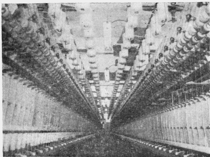
无锡市协新毛纺织染厂1983年引进的意大利毛纺锭
