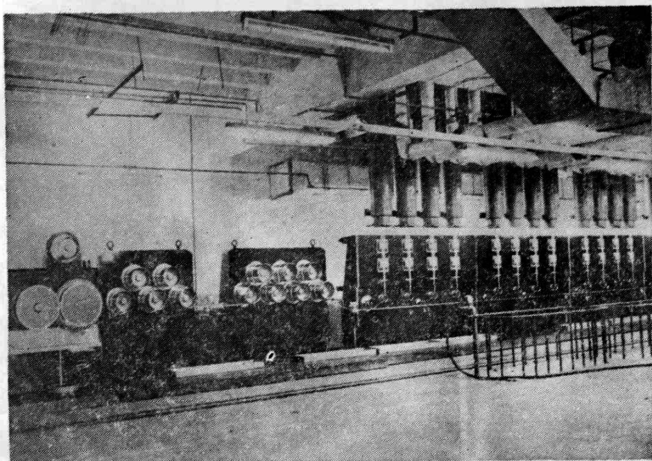
无锡市第二合成纤维厂的多孔短丝纺丝机
