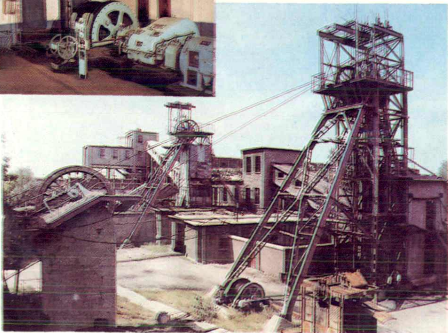
主井、副井(左上图为主井落地摩擦式绞车车房内景)
