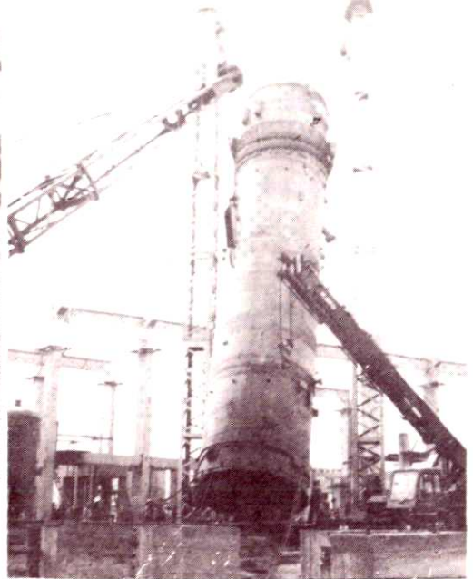
起吊氨合成塔
