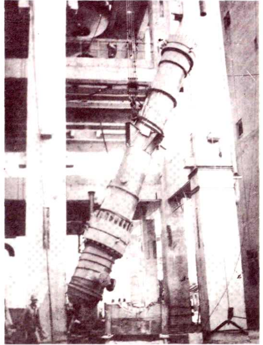
吊装尿素合成塔
