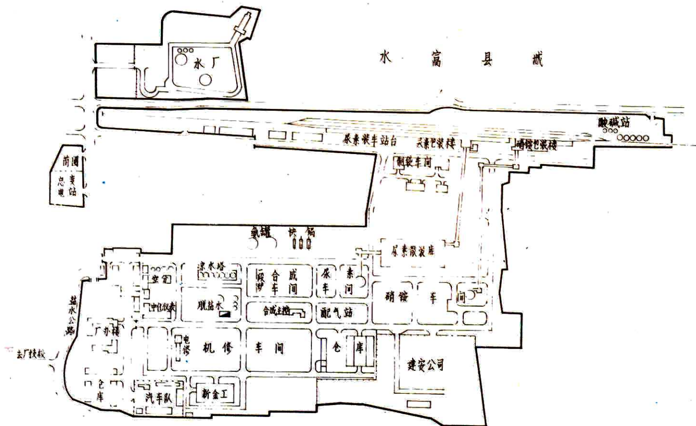
云南天然气化工厂界区平面佈置图
