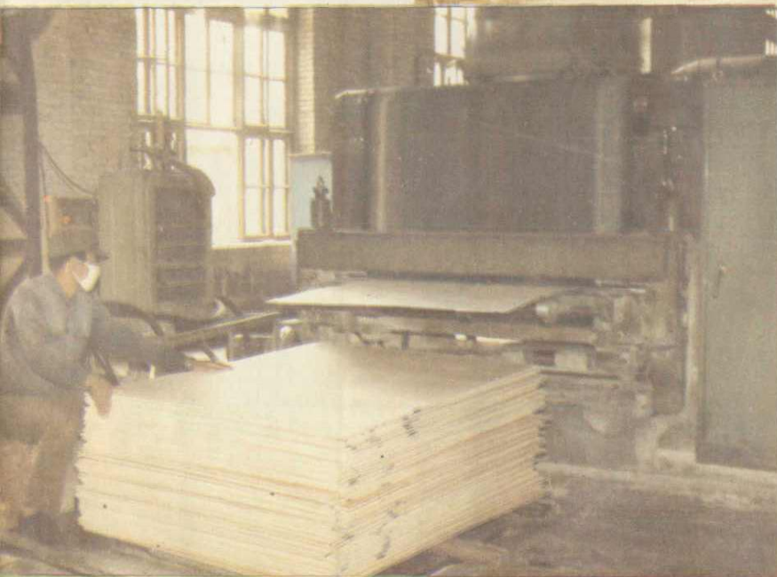
胶合板砂光机
