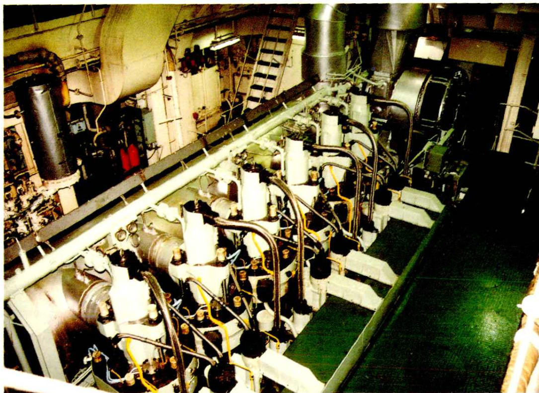
整洁明亮的振奋型货轮机舱
