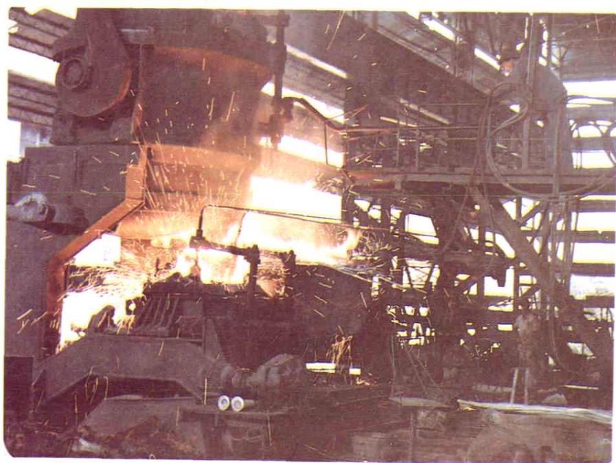
国家计委、冶金部“七五”期间重点攻关项目——不锈钢连铸，由江西钢厂，上钢五厂、上海钢铁工艺技术研究所共同合作，于1986年9月在江钢大方坯连铸机上试验，取得成功。
