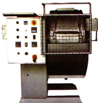
实验转鼓
