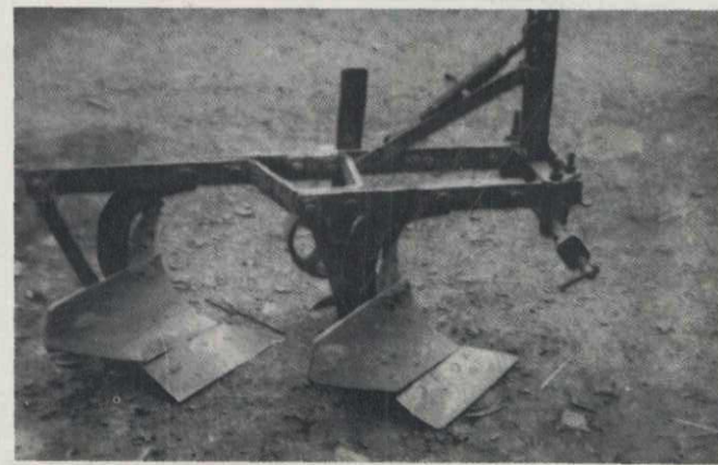
悬挂单向双铧犁
