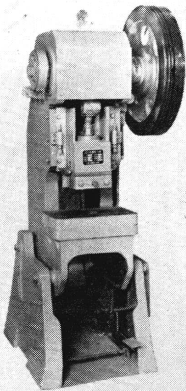
丁23型16吨可倾压力机
