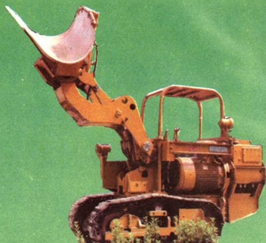
ZCY-60型正装侧卸液压装岩机
