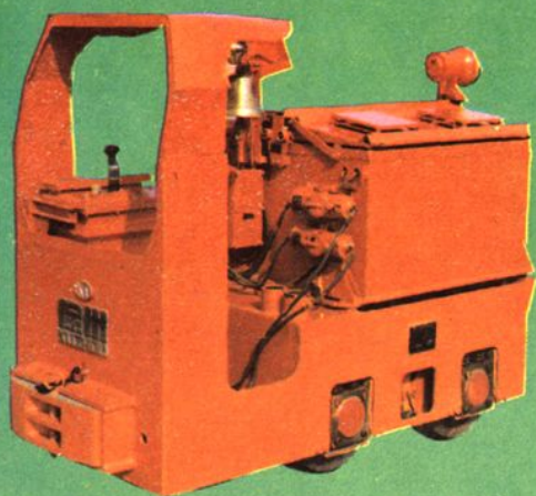
CDXT-2.5矿用隔爆特殊 型蓄电池电机车
