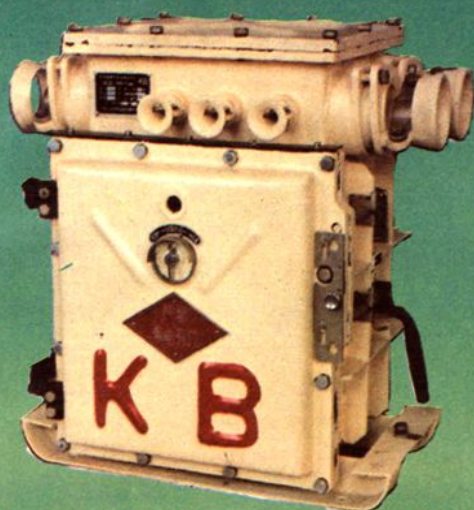
DKZB—400/1140型真空馈电开关
