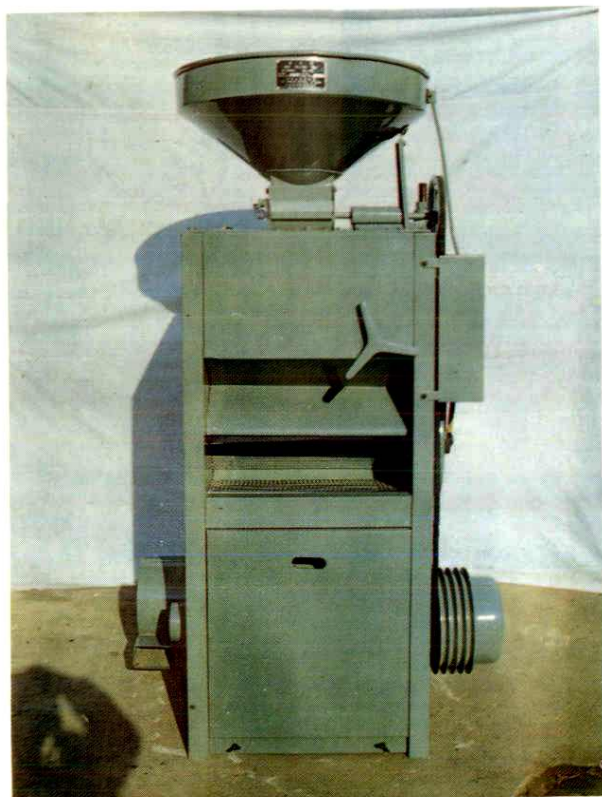
鱼台县机械厂生产的出口产品联合米机
