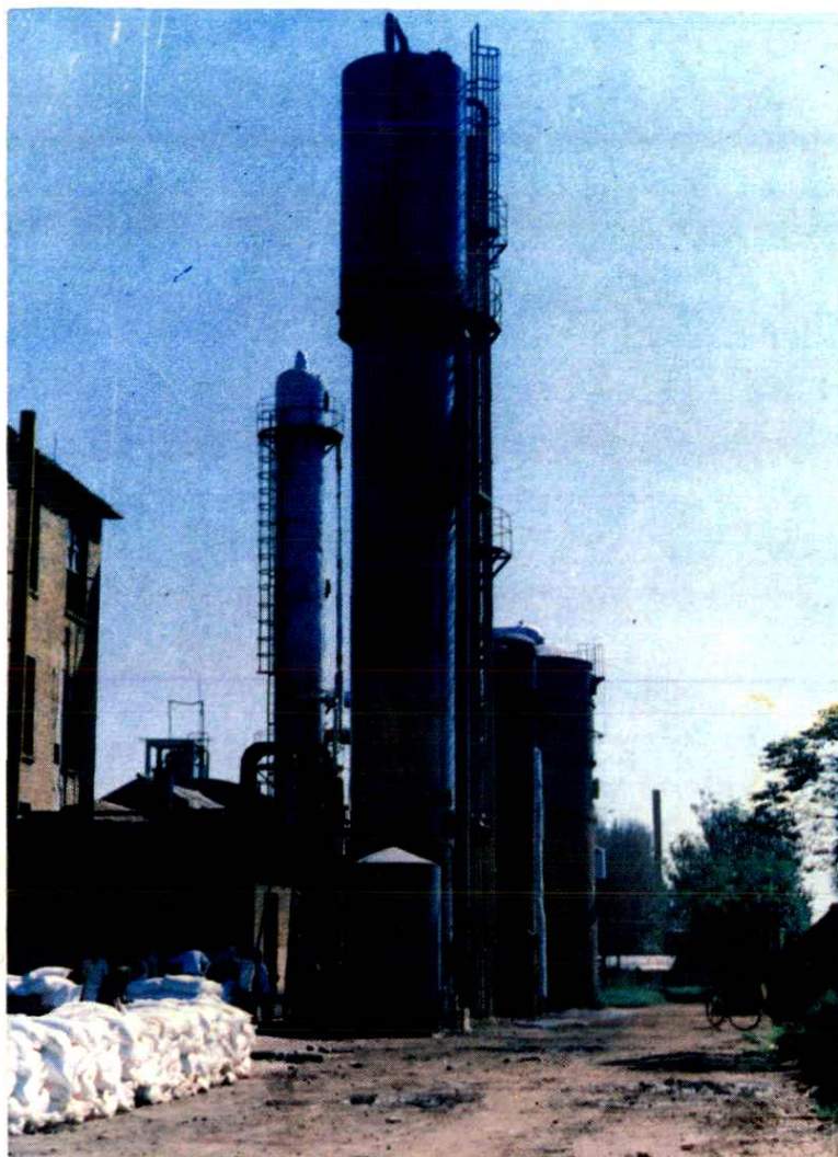
鱼台县化肥厂的生产设施
