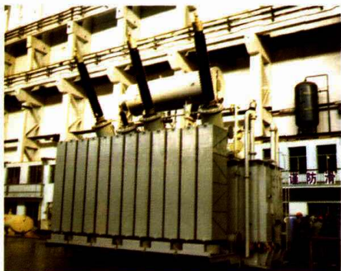
SFPS9-150000/220三相三绕组油浸风冷无励磁调压电力变压器 (带油泵)
