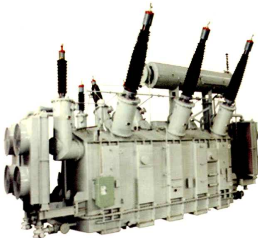
SFPSZ10-150000/220三相三绕组强油风冷有载调压电力变压器
