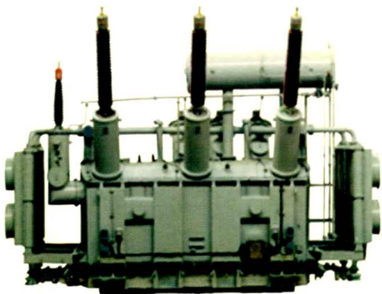
SFP10-240000/220 三相双绕组强油风冷无 励磁调压电力变压器
