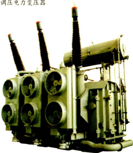
SSZ10-50000/220三相三绕组油浸自 冷有载调压电力变压器
