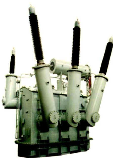
SFP10-50000/220三相双绕组强油风冷 无励磁调压电力变压器
