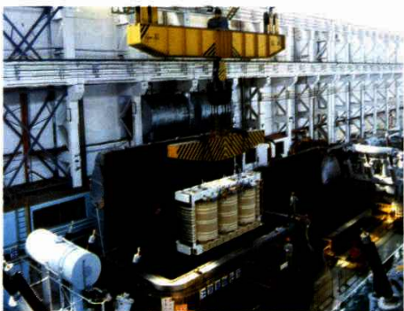
从瑞士麦格菲尔公司引进的400KW煤油气相干燥设备
