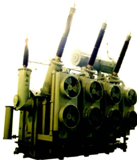
SFPS10-120000/220 三相三绕组强油风冷无 励磁调压电力变压器
