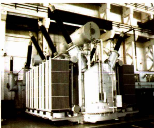
SFS10-180000/220三相三绕组油浸风冷无励磁调压电力变压器
