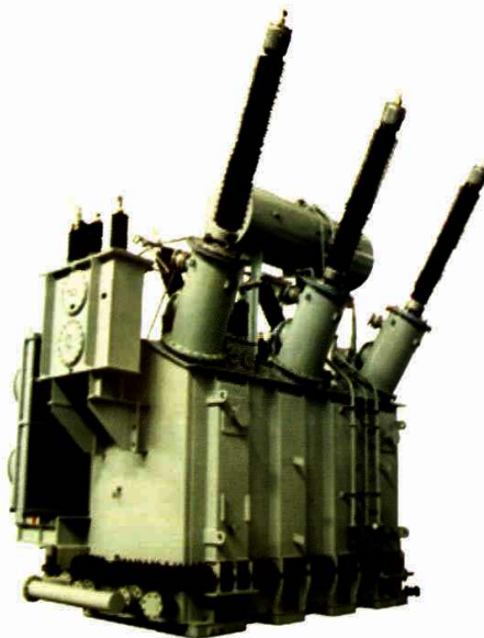
OSFPS10-120000/220三相三绕组自耦强油风冷无励磁调压电力变压器。
