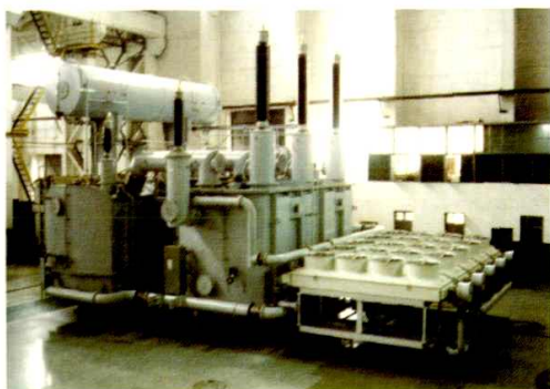
ZHSFPTB-112000/220 三相自耦有载调压整流变压器
