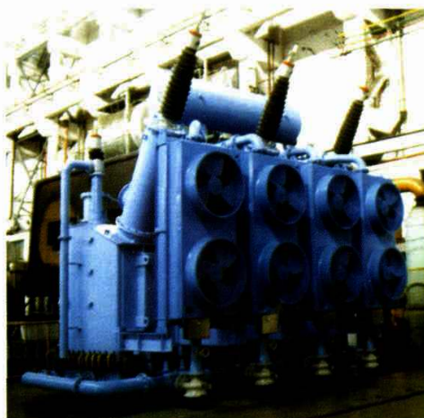
SFSZ10-31500/110 三相三绕组油浸风冷有载调压电力变压器
