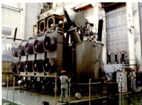
SFPS10-370000KVA/220KV三相双绕组强油风冷无励磁调压电力变压器
