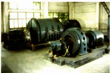
用于变压器试验的15000KVA发电机组
