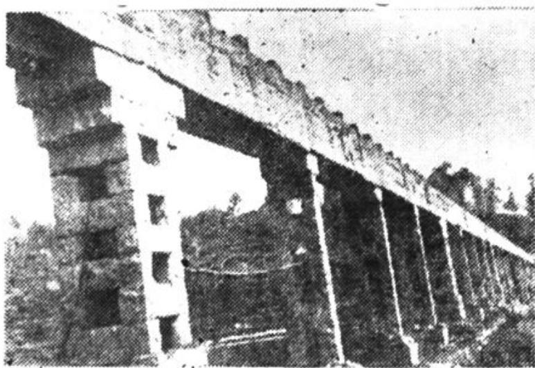
圳口水库天桥。
