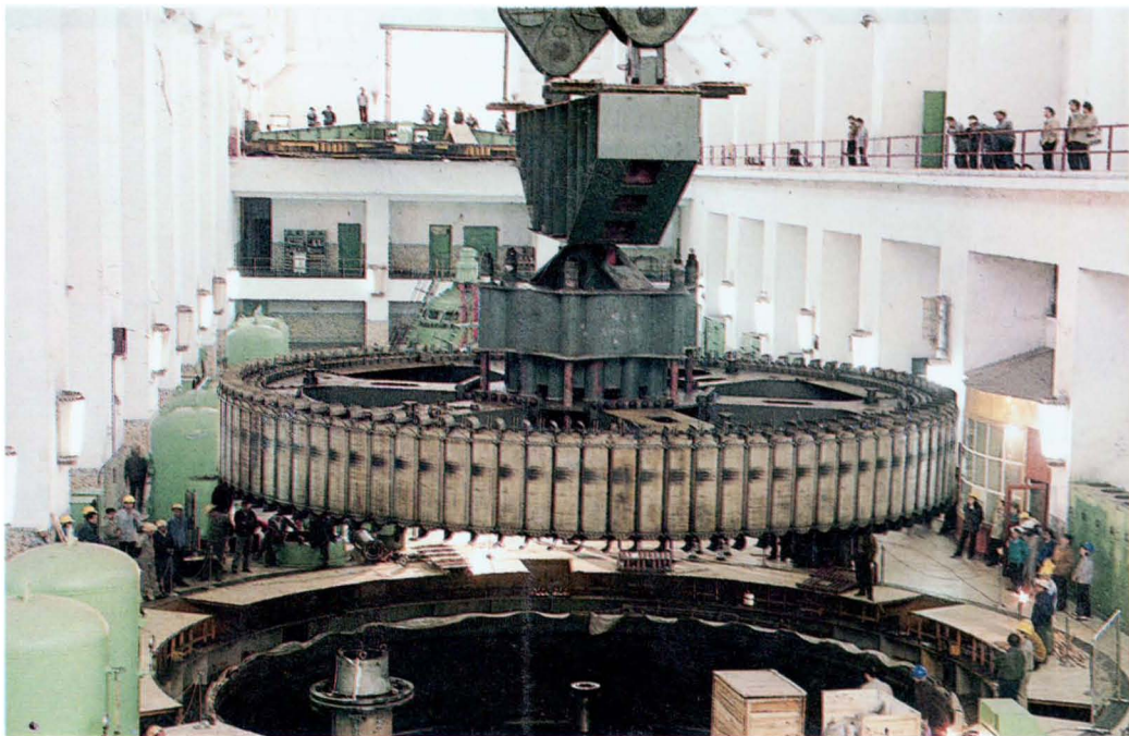
△ 吊装发电机转子(秦昌展摄)
