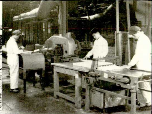
1932年建造的香皂车间切块、自动撞印机
