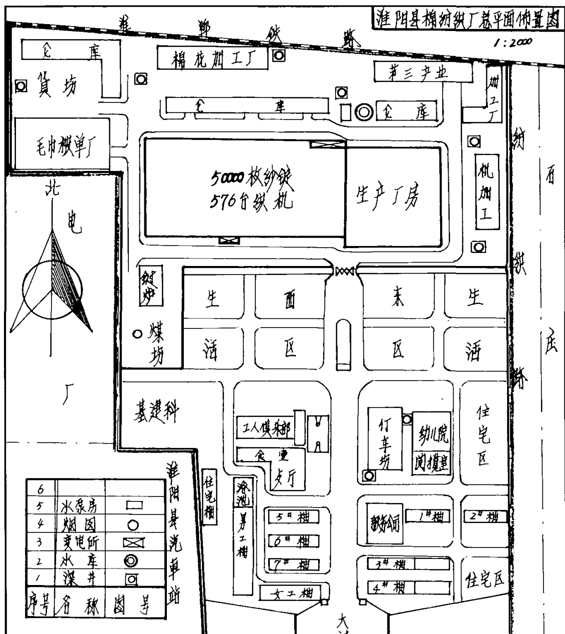
淮阳县棉纺织厂总平面布置图
