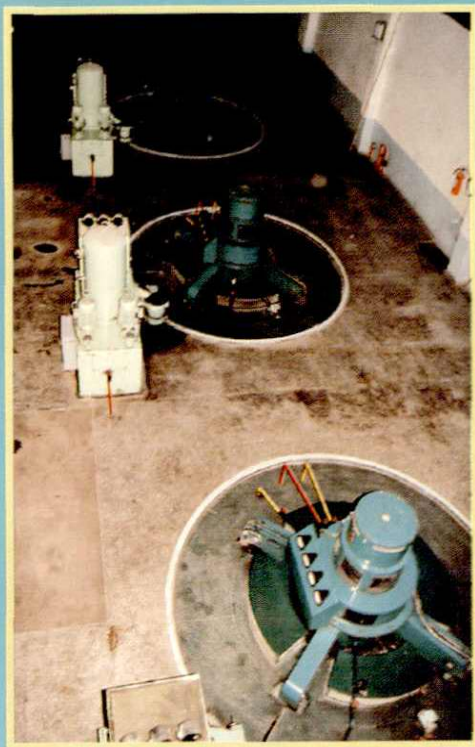
运行中的赤壁电站机组
