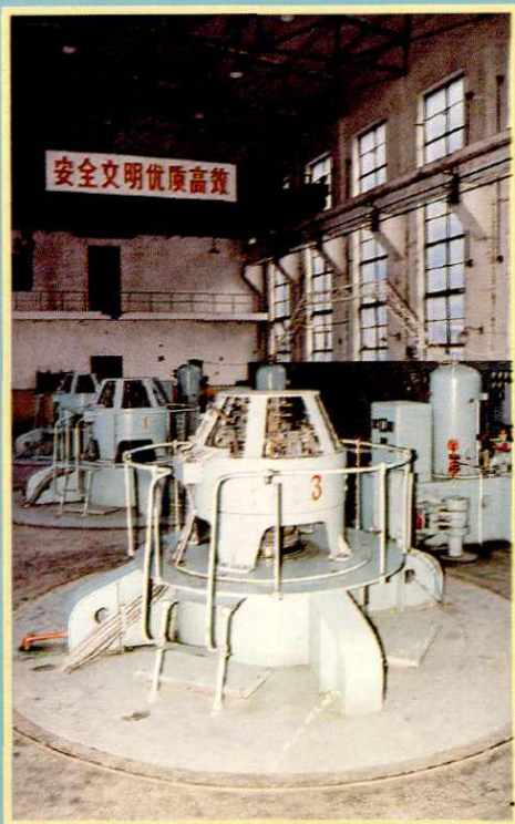
侯壁电站运行机组
