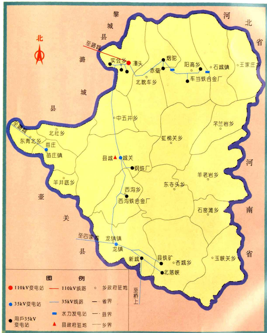
平顺县1996年地理主接线示意图
