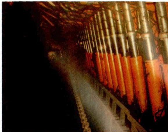
井下综采工作面
