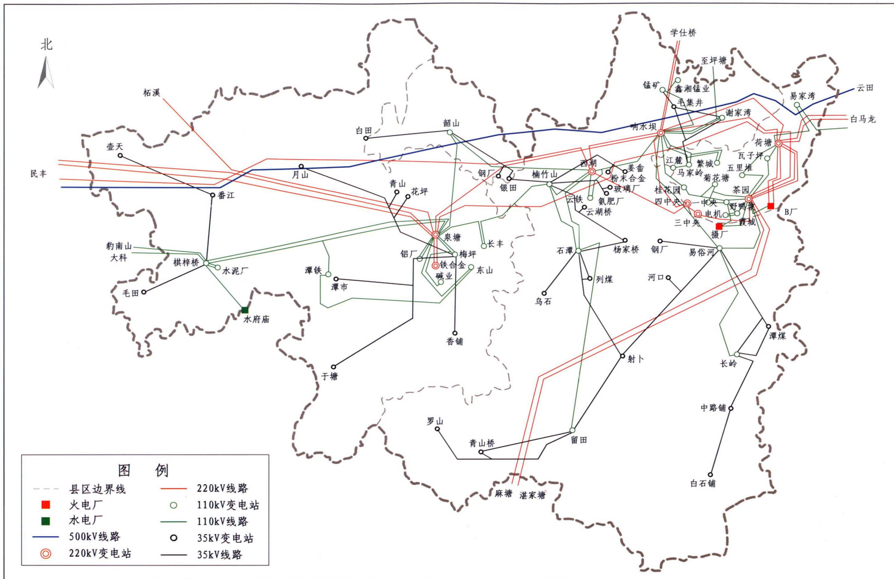
湘潭地区电网2005年地理接线图
