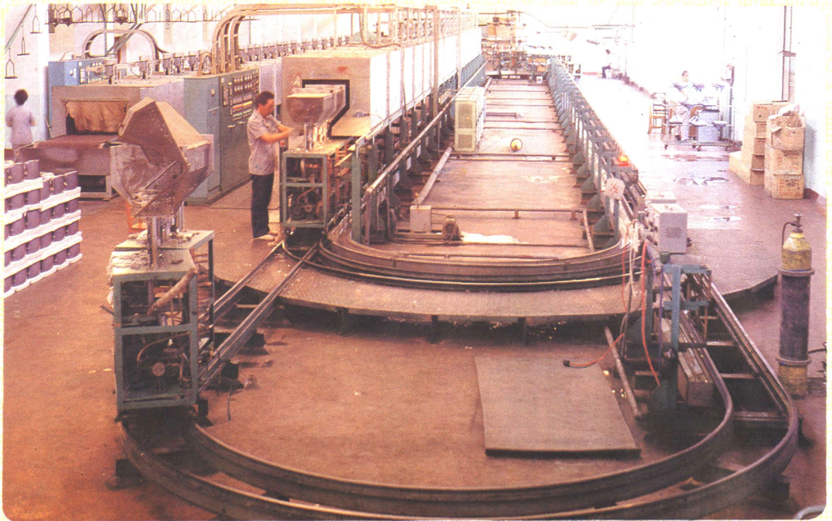
黑白顯象管生產綫在運行
