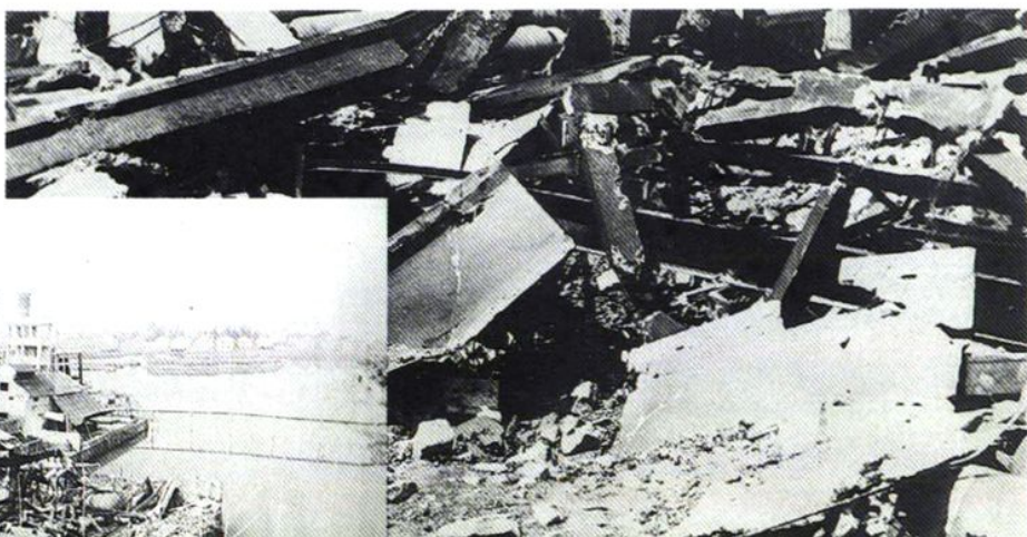
温州电化厂氯气爆炸现场 （温州电化厂供稿）
