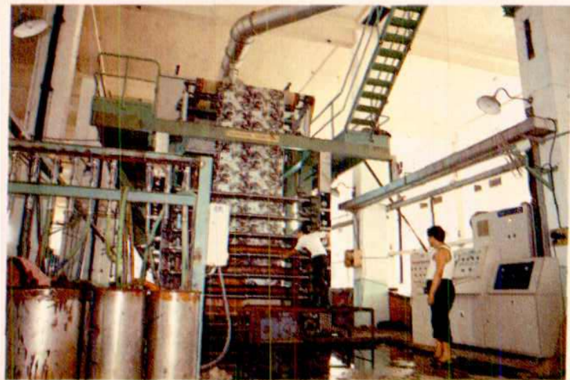
武汉印染厂的双面印花设备。
