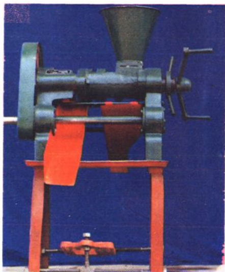
公安县农机修造三厂生产的 小型螺旋榨油机
