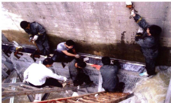
2003年9月上旬汉江发生秋汛，新沟闸新安装的闸门严重漏水翻水，图为出险、抢险现场。
