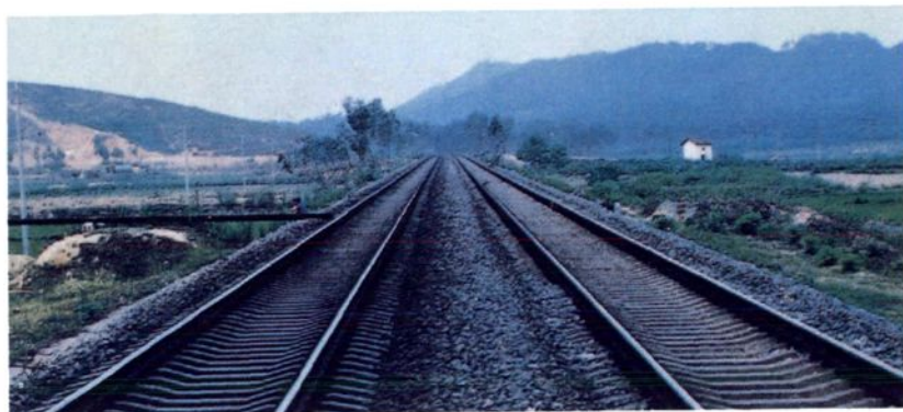
柳黎复线维都至来宾段7.8千米线路
