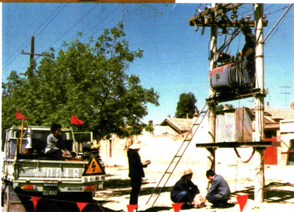
配电变压器现场试验
