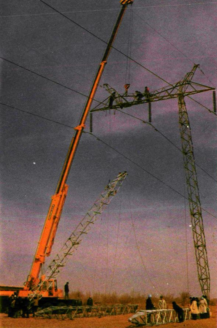
输电线路抢修
