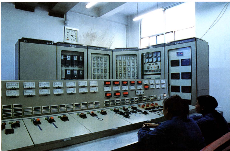
发电厂主控室监测系统
