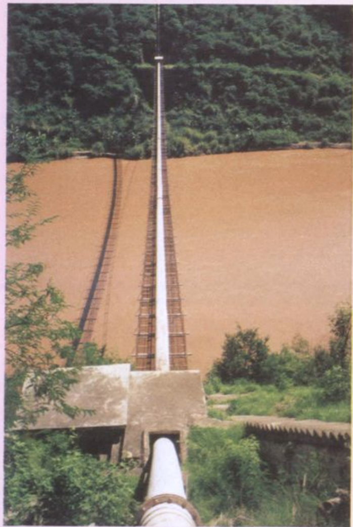
西水东调倒虹吸管
