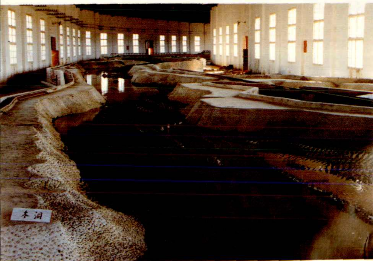
航道水工模型
