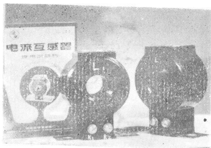
LMK——0.5型75/5A电流互感器
