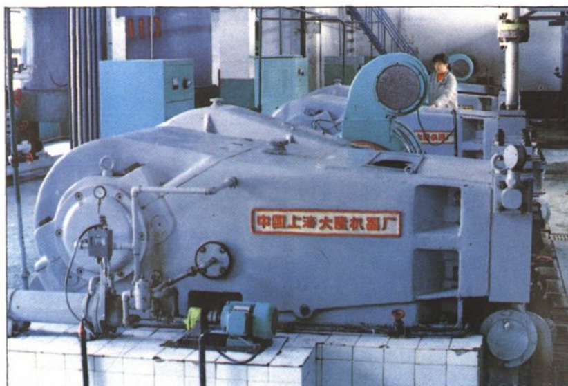
高壓泵泵房
