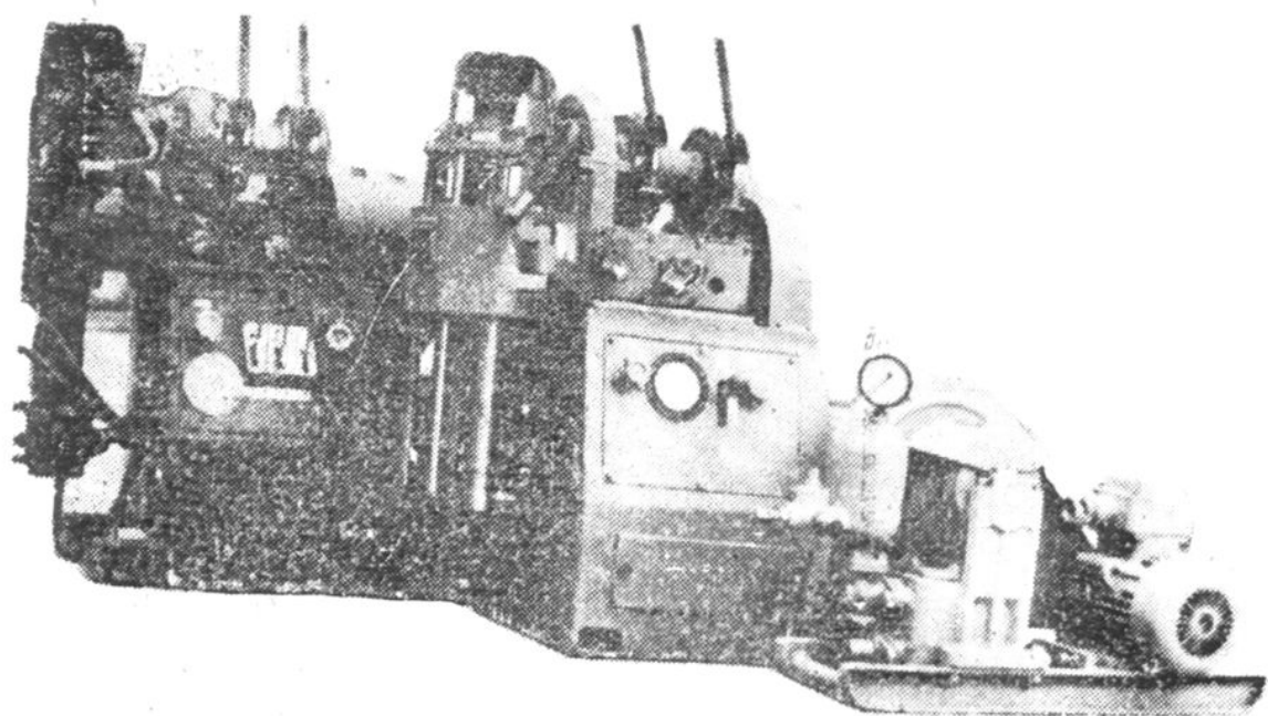
△学院工厂生产的液压钻机和泥浆泵
