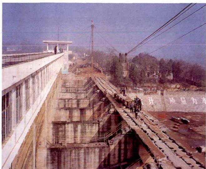
溢洪闸改建工程施工现场
