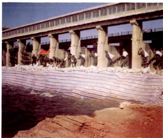
溢洪闸改建工程围堰抢筑
