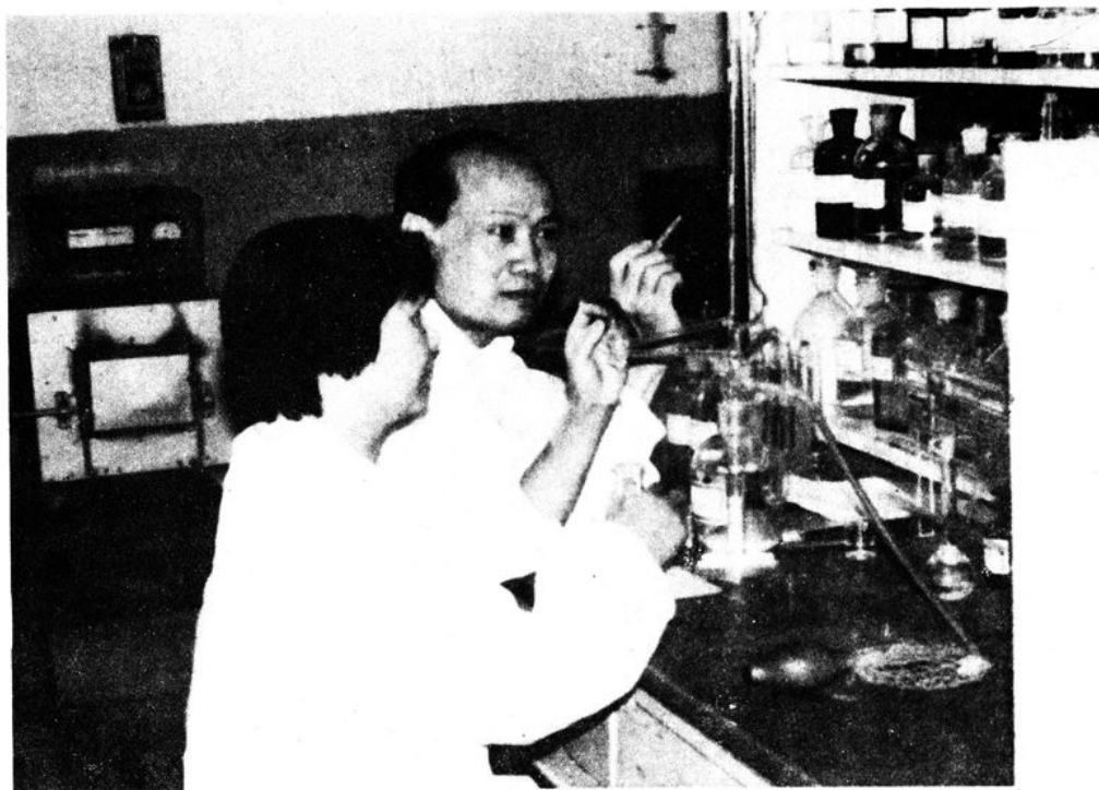
滴 定 操 作
