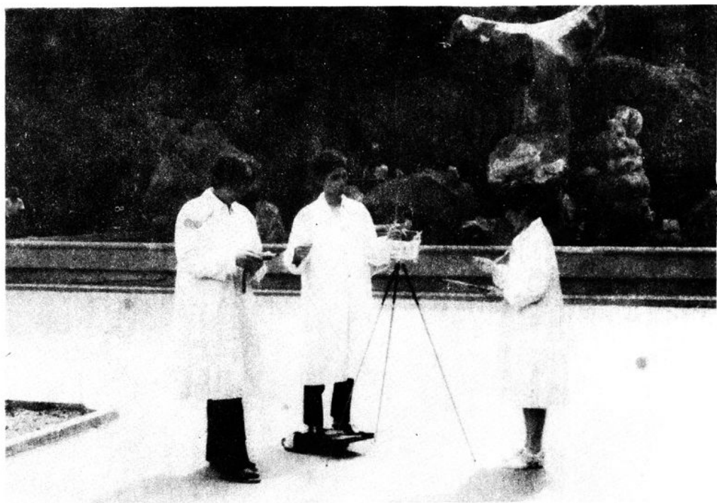
大 气 监 测
