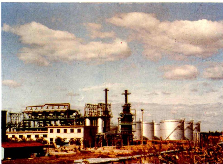
脱蜡装置全景
