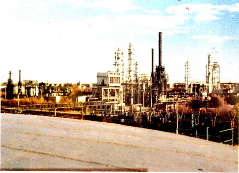
炼油生产装置全景
