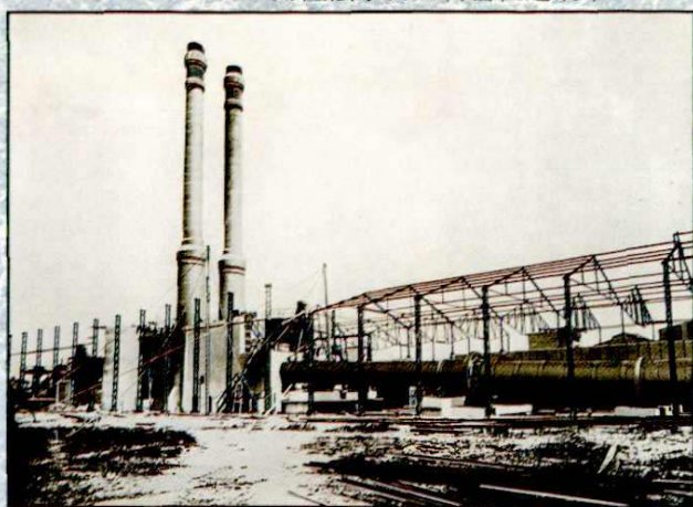
1922年华商上海水泥股份有限公司的湿法水泥回转窑在建设中
