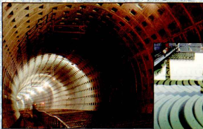
上海水泥制品厂生产的隧道管片用于延安东路越江隧道
