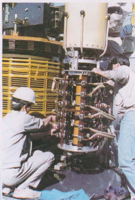
15 主变压器在安装中
