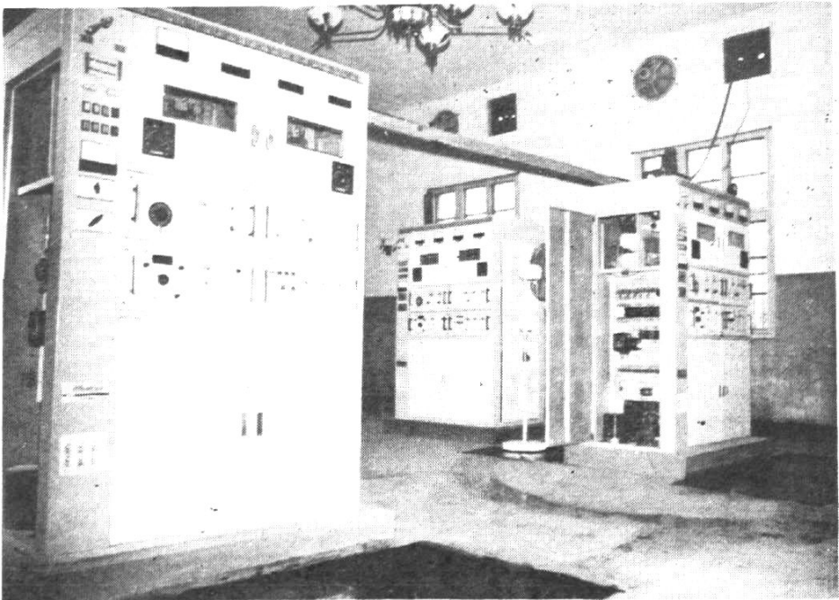
电台中波发射机
