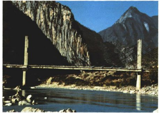
金沙江其春大桥
