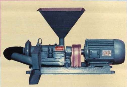
微型碾米机
