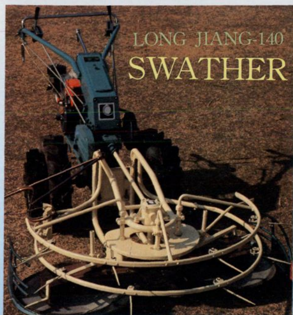
龙江-140 型圆盘式收割机
