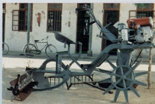
水田耕作机
