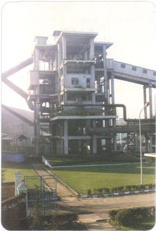
8 平方米球团竖炉
