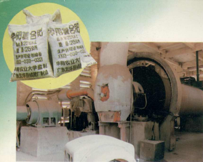
• 縣磷肥廠生產磷肥的主要機械及其產品 •
