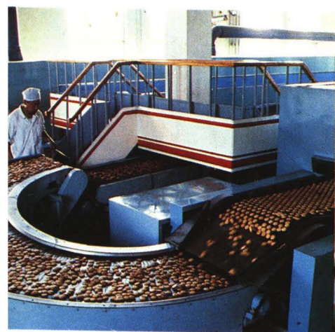
北京第一食品厂饼干生产线
