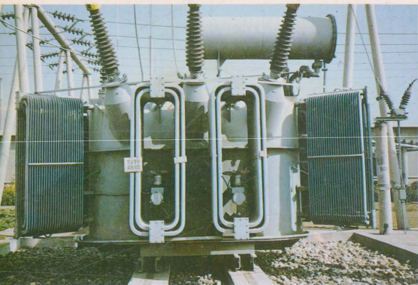
十一万变电站1号主变
