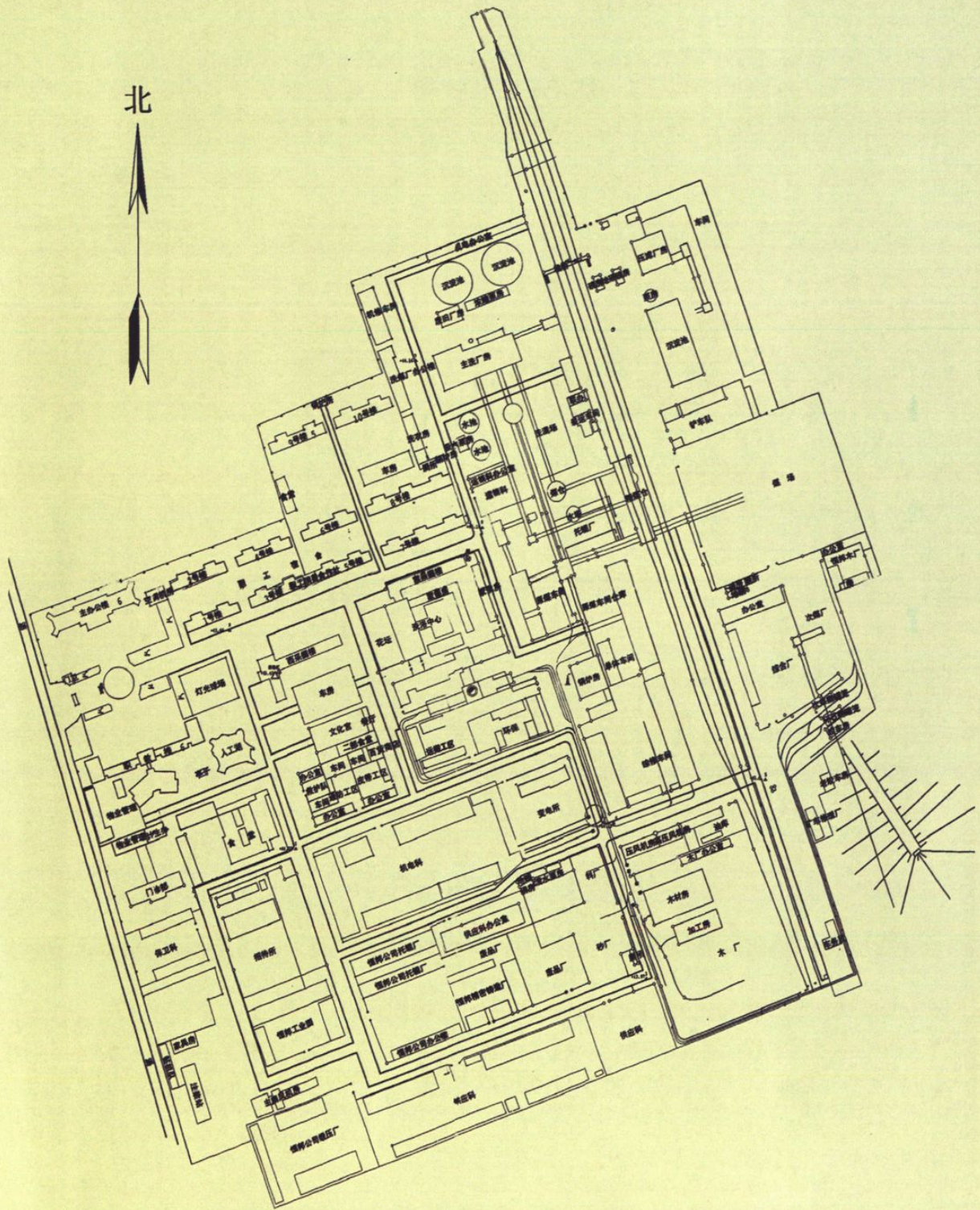
田陈矿工业广场平面图
