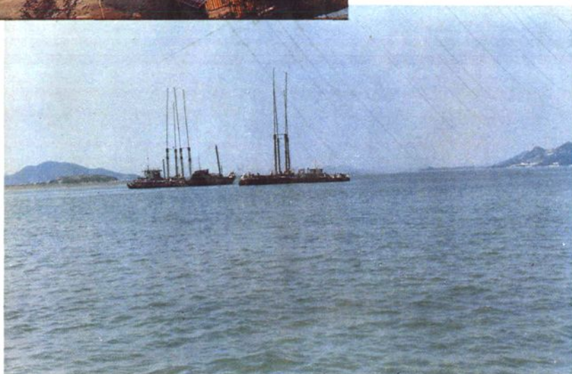
过桥山围垦工程软基础处理： 水上打设塑料排水带
