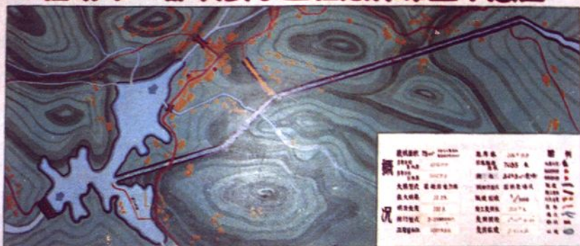
▲ 一都溪引水工程总体布置示意图
