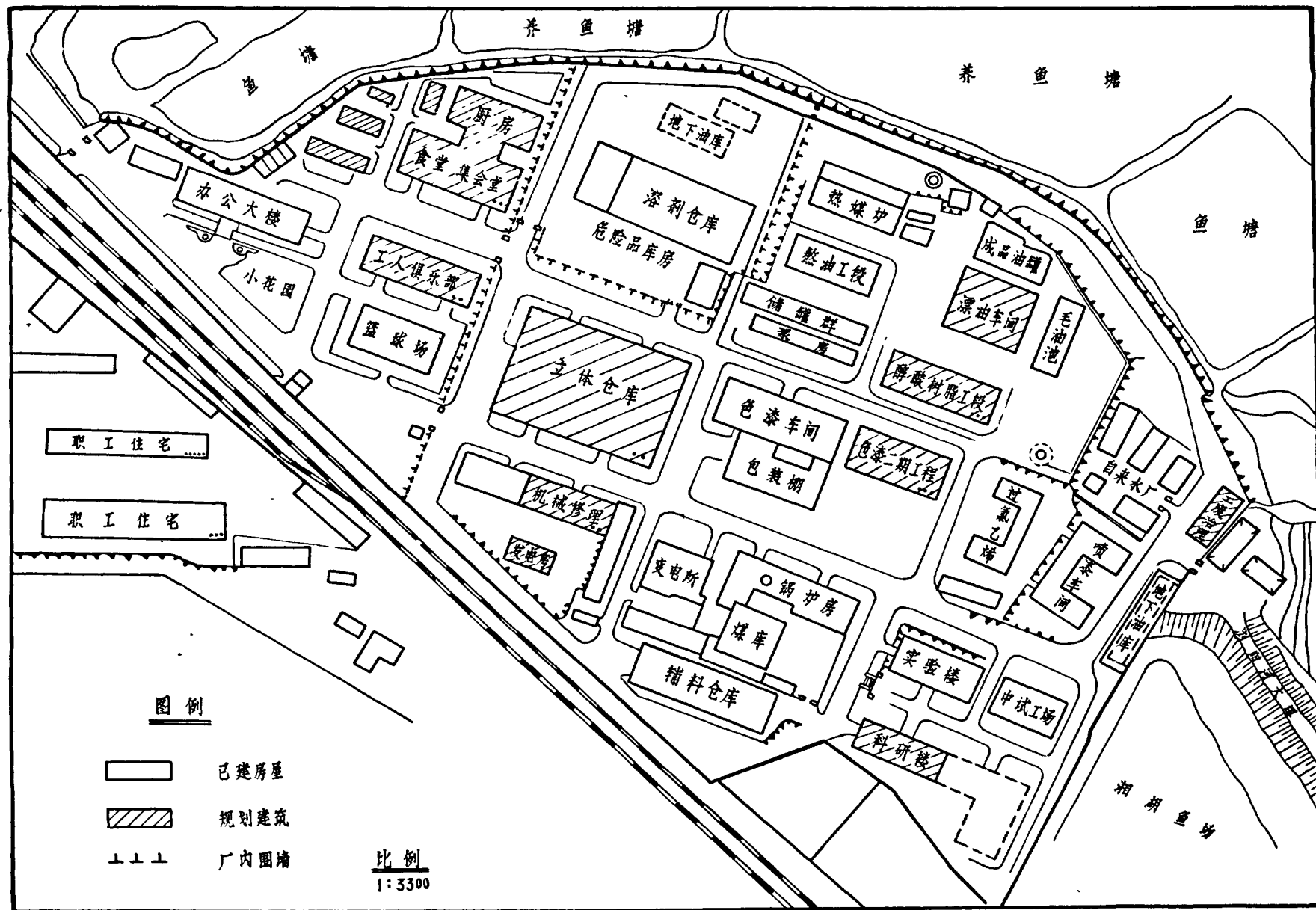
湖南造漆厂平面布置图(南厂区)
