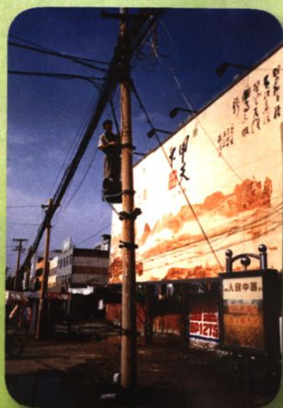
机线员杆上作业
