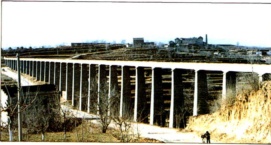
北留水轮泵站北村渡槽
