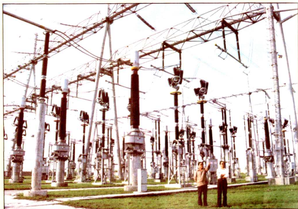
淮南平圩发电厂50万千伏电力升压站
